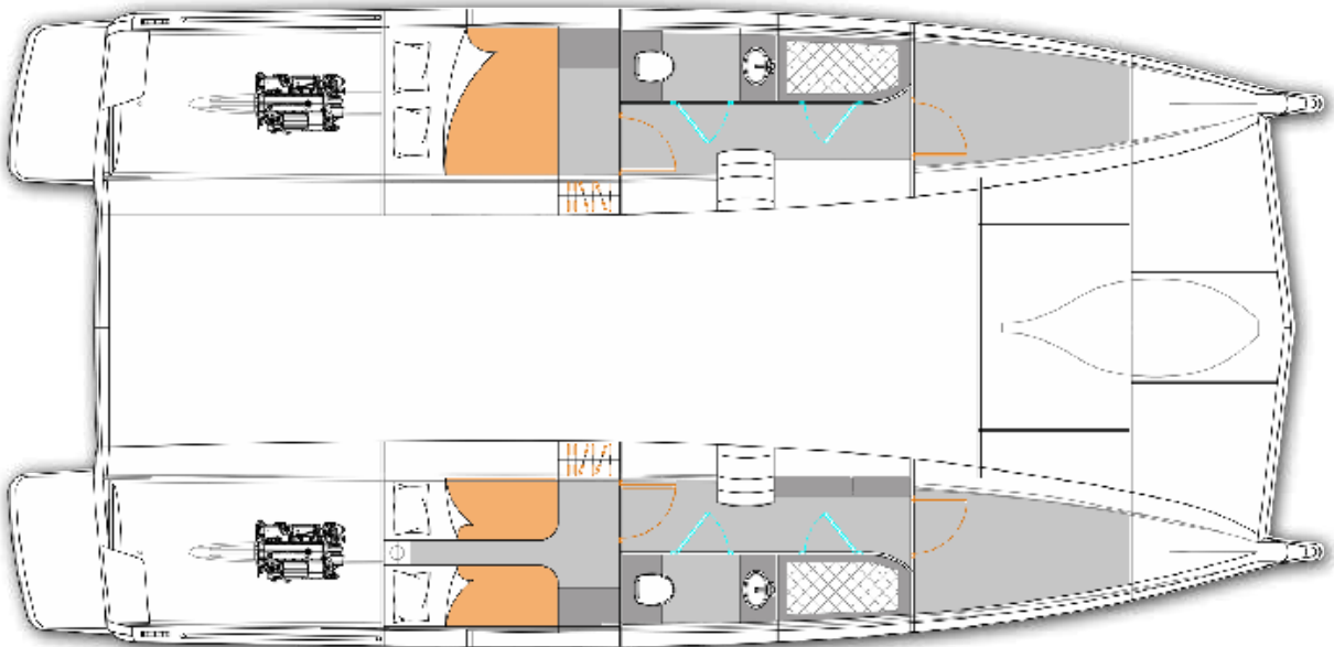
แปลนพื้นที่ ตัวเรือ 2 ห้องนอน- 2 ห้องน้ำ - 2 ห้องอาบน้ำ - 2 ห้องเก็บของ
