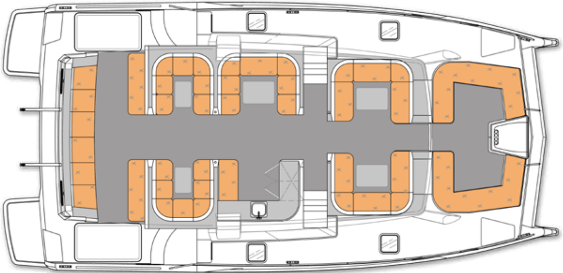
แปลนพื้นที่ ดาวฟ้าหลัก ตั้งแต่หัวเรือจรดท้ายเรือ
