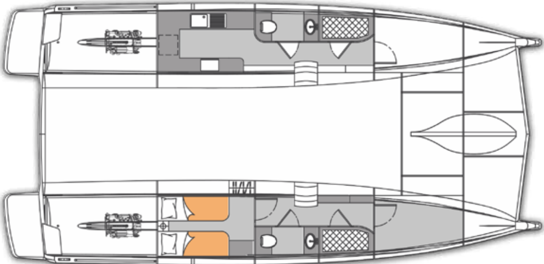
แปลนพื้นที่ ตัวเรือ ห้องนอน-ห้องครัว - 2 ห้องน้ำ - 2 ห้องอาบน้ำ - 2 ห้องเก็บของ
