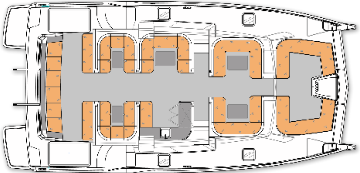
แปลนพื้นที่ ดาวฟ้าหลัก ตั้งแต่หัวเรือจรดท้ายเรือ
